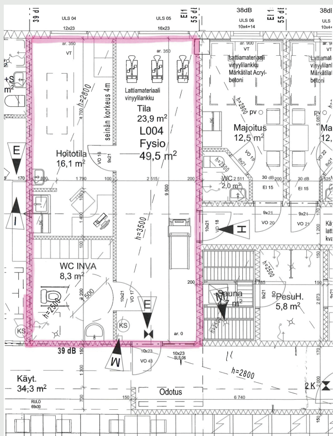
Pohjapiirros
